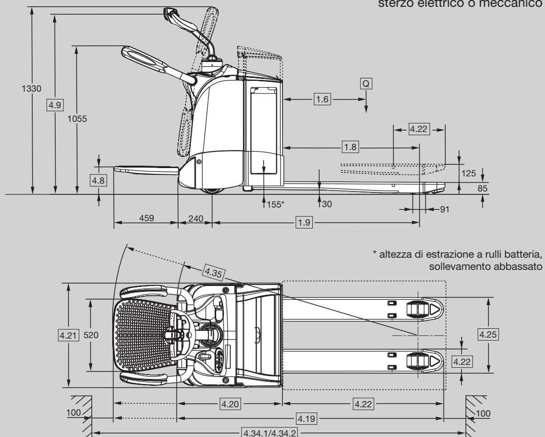
WT 3040-2.0 piattaforma richiudibile, sterzo elettrico o meccanico
